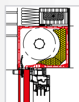
Pose en double mur
