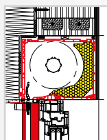
Pose en isolation thermique extérieur
