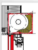
Pose en applique isolation 100 mm
