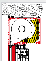
Pose en applique sous dalle
